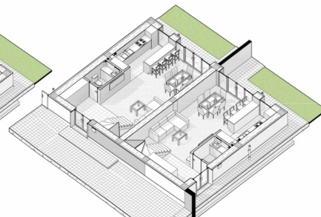
Bloc A - Parter PLANIMETRIE PROPUȘĂ
