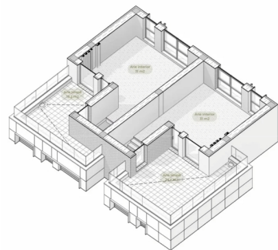
Bloc A - Parter + 2E PLANIMETRIE LIBERĂ
