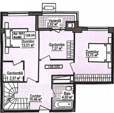
Plan Etaj 10. la cota 30.000
