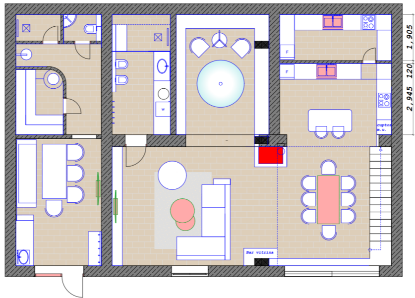
Plan Amenajare Mobilier-Demisol
