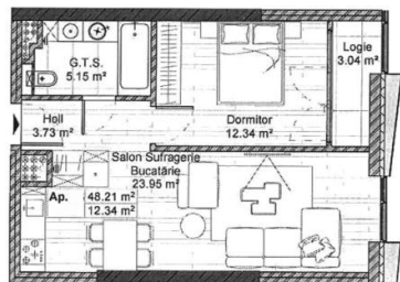
Schema amplasarii apartamentului la etaj
